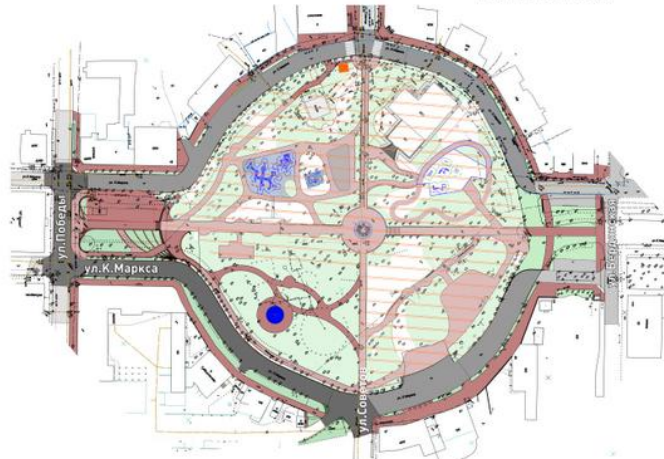
ГЕНПЛАН М 1:500
